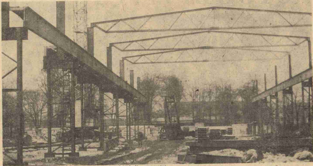
Montaż konstrukcji hali naprawczej
