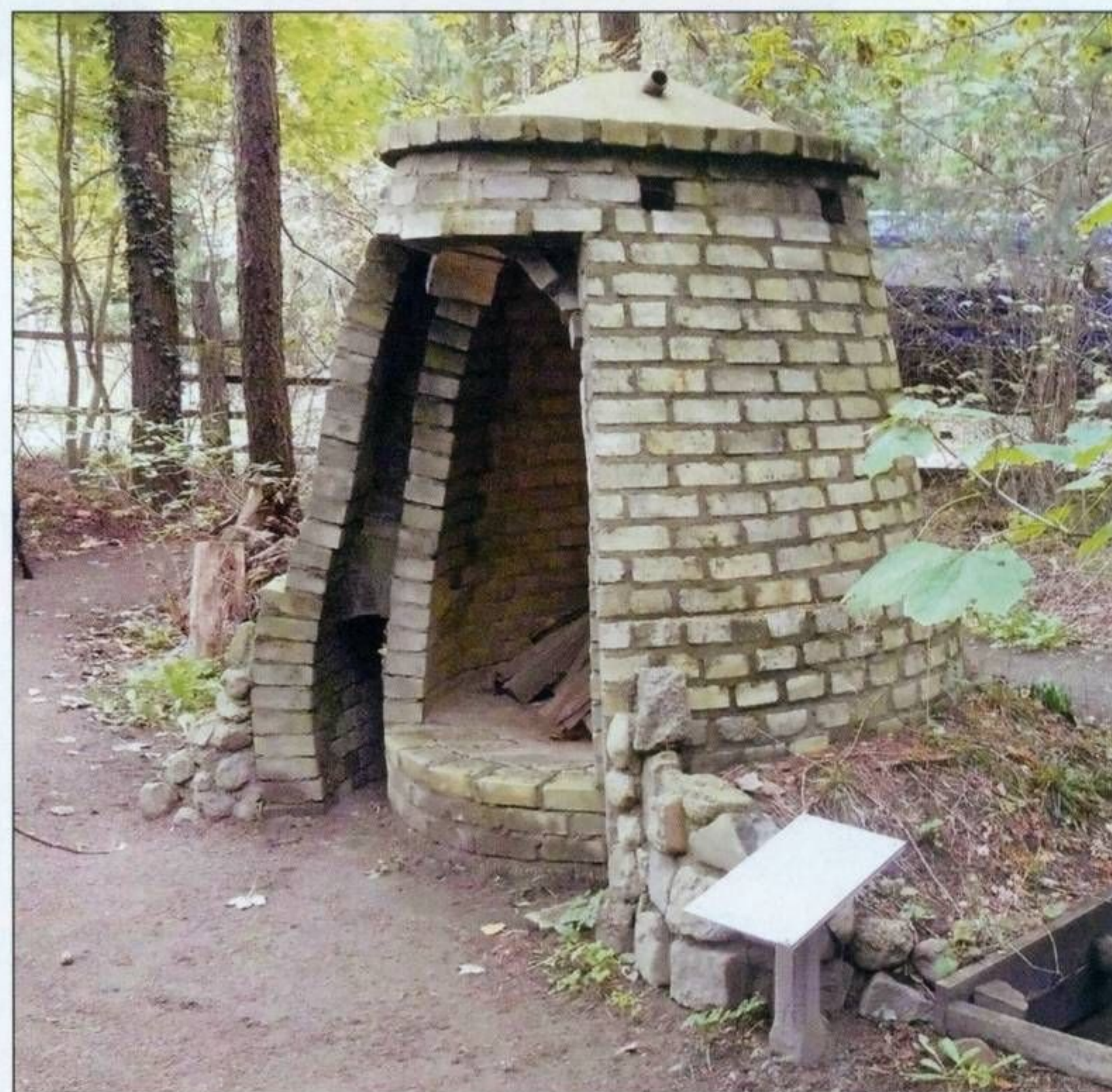
Anschauungsmodell eines kleinen Teerofens im Schnitt, zu sehen im Freilichtmuseum Rövershagen-Wiethagen. (JU)
