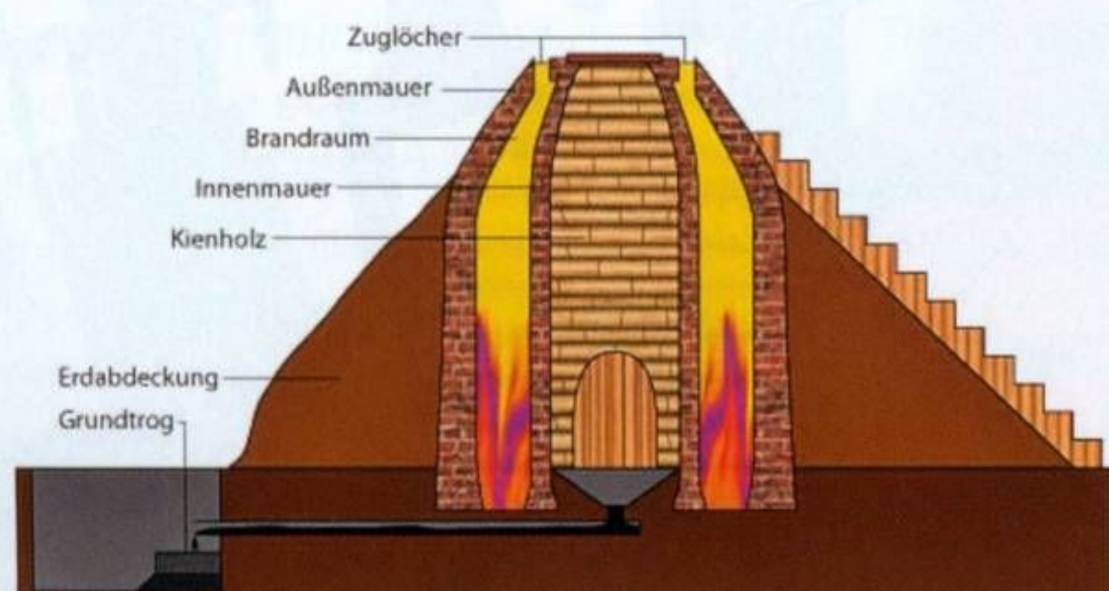
Schnittbild durch einen Teerofen.
